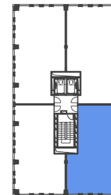
PÔDORYS 8.NP
