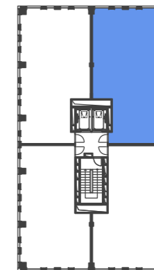
PÔDORYS 7.NP
