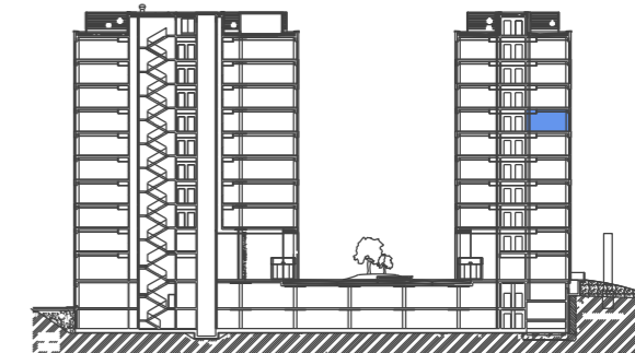
POZDĽŽNY REZ OBJEKTOM DUETT I. DUETT II.
