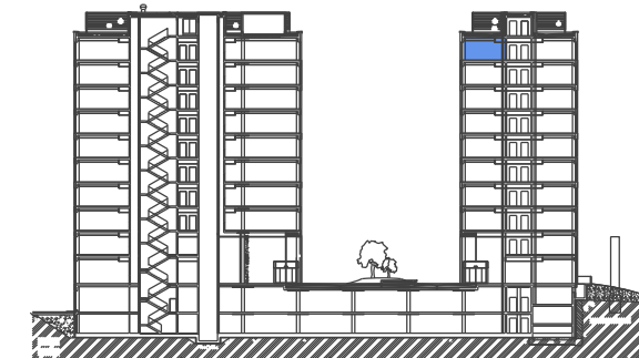
POZDĹŽNY REZ OBJEKTOM DUETT I. DUETT II.
