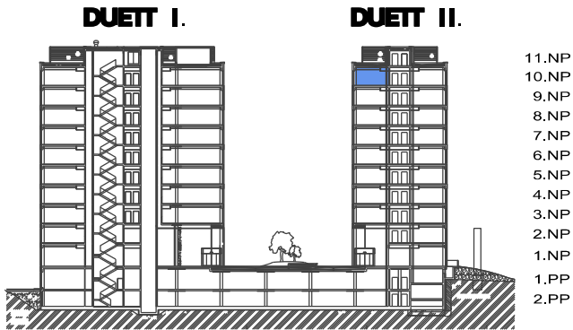
POZDĽŽNY REZ OBJEKTOM
