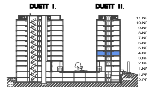
POZDĽŤNY REZ OBJEKTOM
