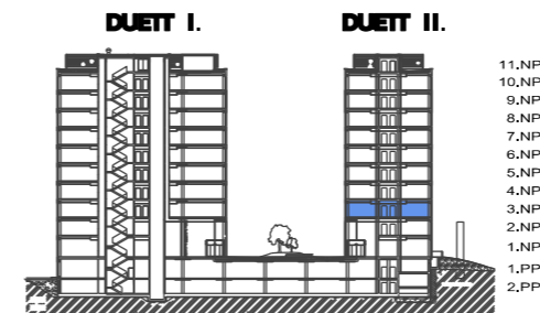
POZDĽŽNY REZ OBJEKTOM
